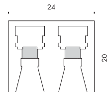
montantelettrico ma2 scala · scale 1:1
