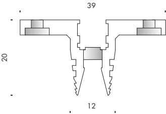
montantelettrico mb1 scala · scale 1:1
