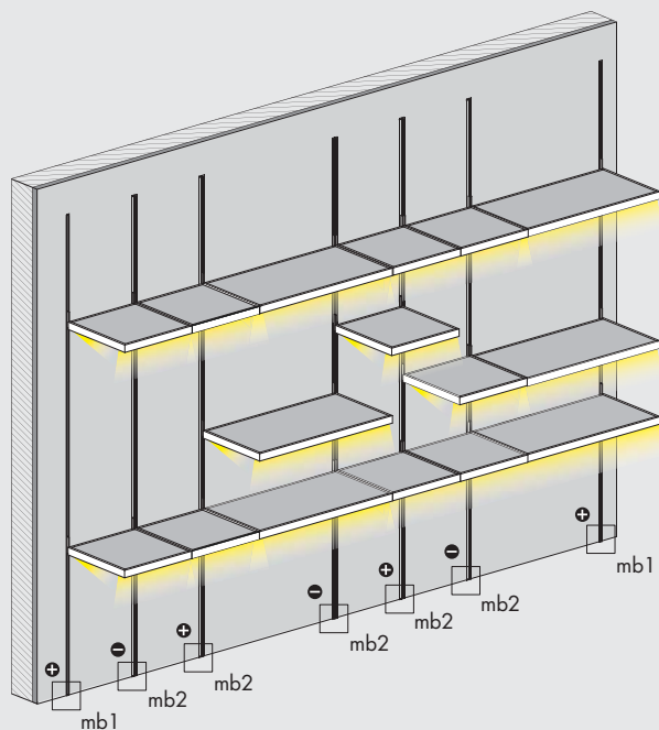
collegamento elettrico · electrical connection montantelettrico mb1
