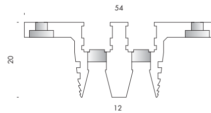
montantelettrico mb2 2000/3000mm scala · scale 1:1
