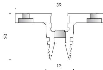
montantelettrico mb1 2000/3000mm scala · scale 1:1
